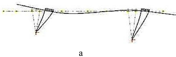
Рис. 1. Основные формы собственных колебаний перегружателя:
