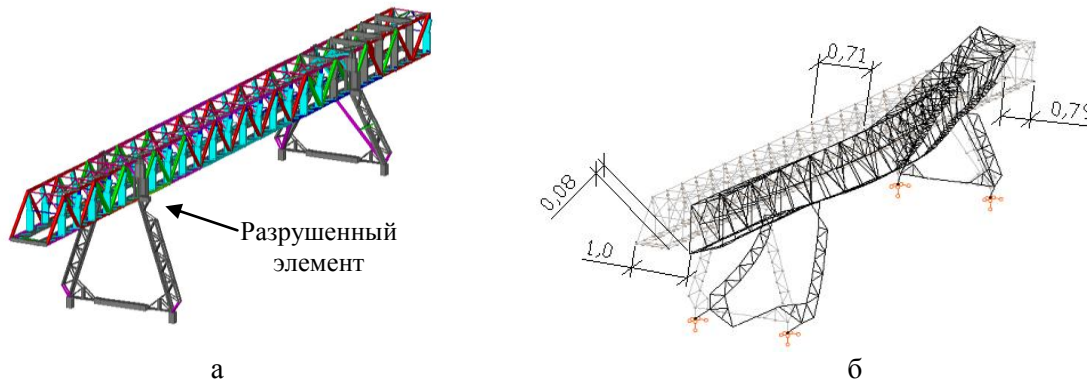
Рис. 7. Низшая форма собственных колебаний перегружателя с поврежденным элементом гибкой опоры: а – пространственная модель перегружателя с разрушенным элементом гибкой опоры; б – низшая форма горизонтально-поперечных изгибных колебаний моста с закручиванием и смещением гибкой опоры на частоте 0,58 Гц
