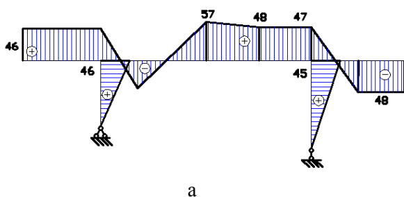
Рис. 2. Эпюры динамических коэффициентов по перемещениям для основных форм колебаний перегружателя:
