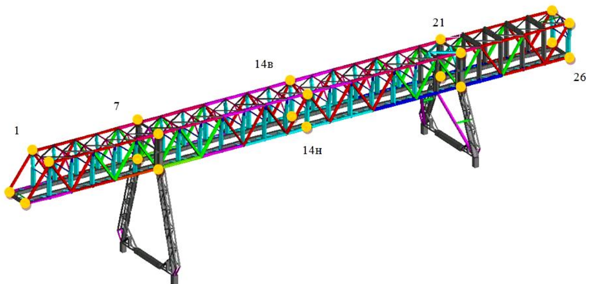
Рис. 4. Пространственная 3-D модель решетчатого перегружателя с приложенными сосредоточенными массами: m.1 - 4 \times 8,78t ; m.7 - 4 \times 39,06t ; m.14в - 4 \times 37,77t ; m.14н - 2 \times (37,77t + 63,9t) ; m.21 - 4 \times 41,24t ; m.26 - 4 \times 10,62t
