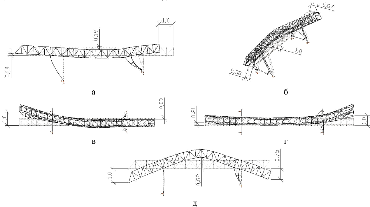
Рис. 5. Схемы собственных колебаний перегружателя: а – 0,61 Гц горизонтально-продольная в вертикальной плоскости; б – 0,62 Гц горизонтально-поперечные изгибные колебания моста с закручиванием и смещением гибкой опоры моста; в – 0,83 Гц горизонтально-поперечные колебания консоли гибкой опоры (вид сверху); г – 1,03 Гц горизонтально-поперечные колебания консоли жесткой опоры (вид сверху); д – 1,72 Гц изгибные вертикальные колебания моста
